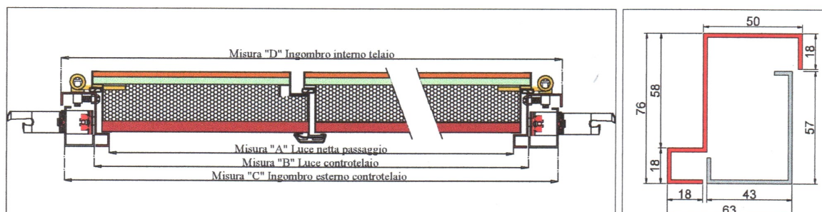
Sezione telaio e controtelaio
